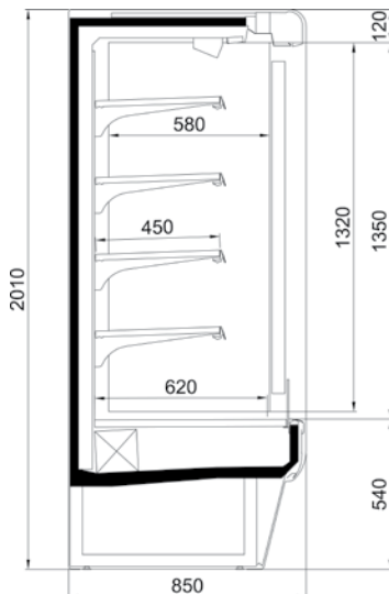
ECO TWIST M2 (Variante) mit bis zu 65% Energieeinsparung zum herkömmlichen Modell Messung nach EN 23953-1
