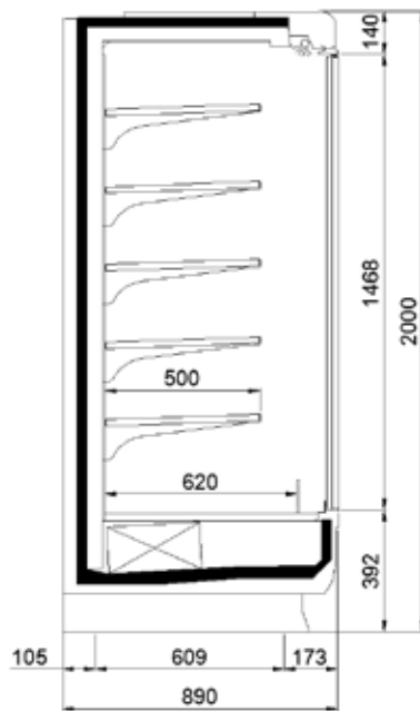
Sonderausführung EURO BALI-T in schwarz mit Full-Vision Türen
