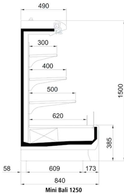
MINI BALI mit Kopfteil Anwendungsbeispiel - auf Anfrage
